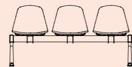
EP15 L 157 x W 60 x H 78 cm
