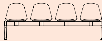
EP16 L 209 x W 60 x H 72 cm
